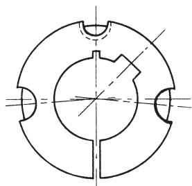
ESECUZIONE A N° 3 FORI
